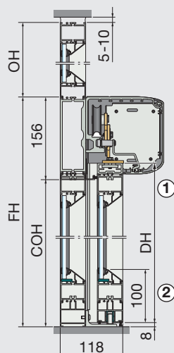
Singola anta con anta laterale e soprauce (apertura verso sinistra in figura)
