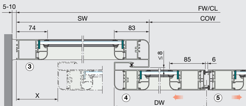
Singola anta senza anta laterale (apertura verso sinistra in figura)
