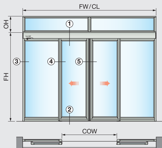
Montaggio a trave, doppia anta con ante laterali e soprauce
