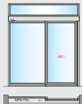
Singola anta con anta laterale e soprauce (apertura verso sinistra in figura)
