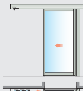
Singola anta senza anta laterale (apertura verso sinistra in figura)
