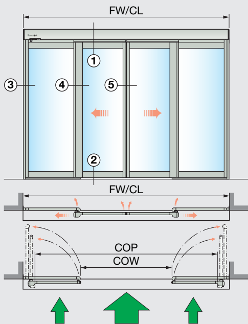
Doppia anta con ante laterali e sistema antipanico, montaggio a muro
