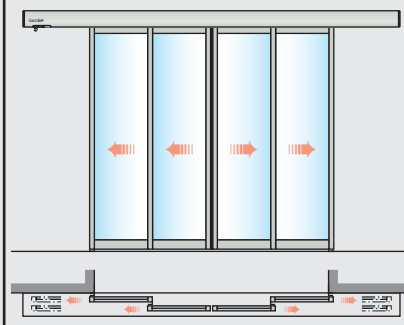
Ante telescopiche a singolo scorrimento con anta laterale fissa (apertura verso sinistra in figura)
