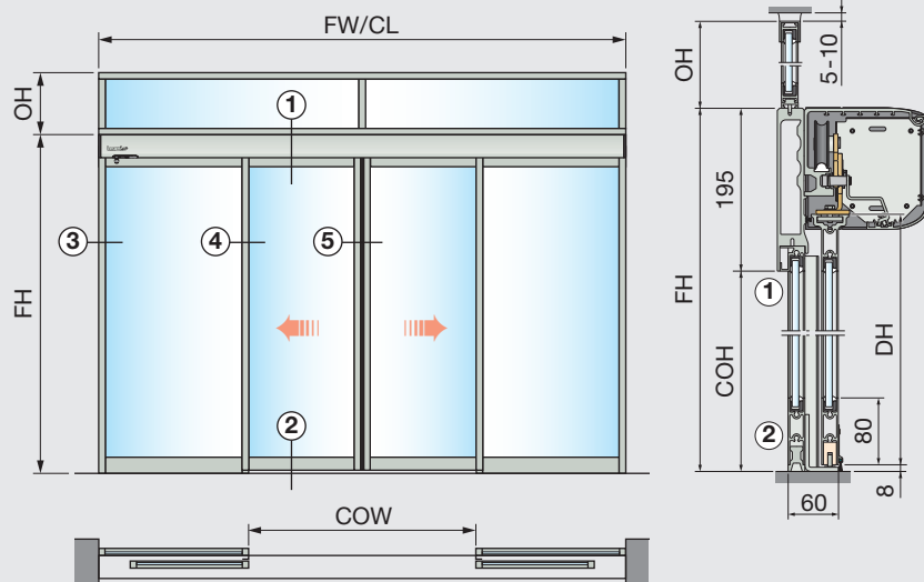
Montaggio a trave, doppia anta con ante laterali e sopra luce
