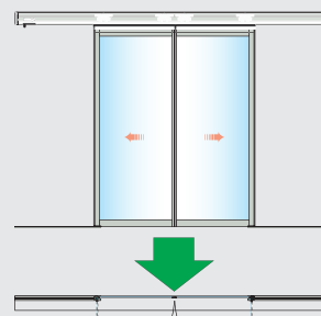
Doppia anta con sistema antipanico senza laterali fissi
