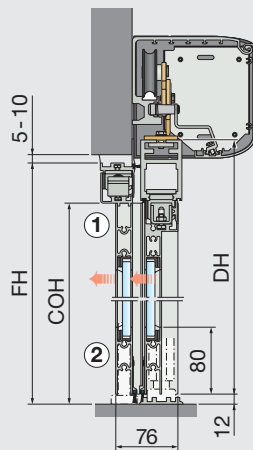
Doppia anta con ante laterali e sistema antipanico, montaggio a muro
