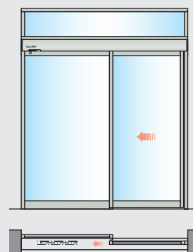
Singola anta con anta laterale e sopra luce (apertura verso sinistra in figura)
