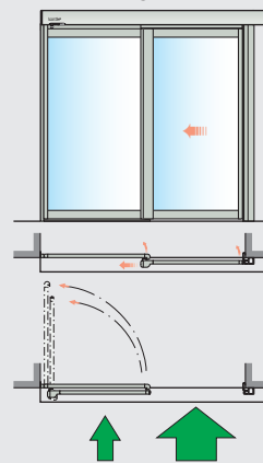
Doppia anta con sistema antipanico senza laterali fissi
