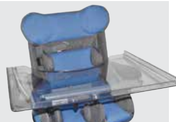
870041 Tavolino con incavo, in plexiglass, con regolazione dell'altezza e dell'inclinazione, ribaltabile.
