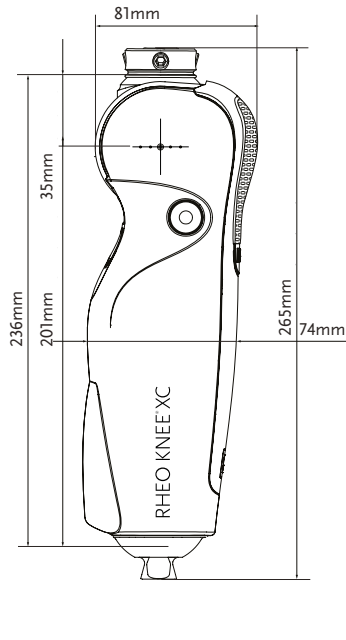
RHEO KNEE XC CON ADATTATORE PER DISARTICOLAZIONE DI GINOCCHIO (A-145310)
