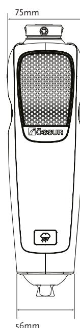
RHEO KNEE XC CON ADATTATORE PER DISARTICOLAZIONE DI GINOCCHIO (A-145310)
